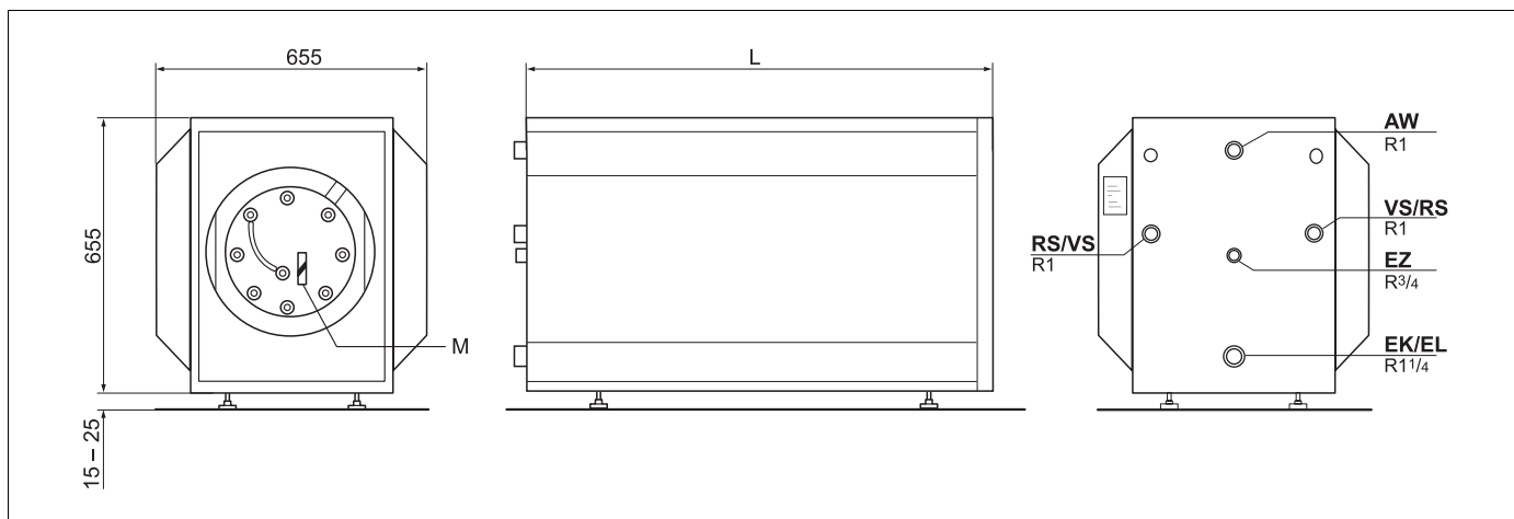
Sl. 2 Dimenzije i priključci (mjere u mm)
