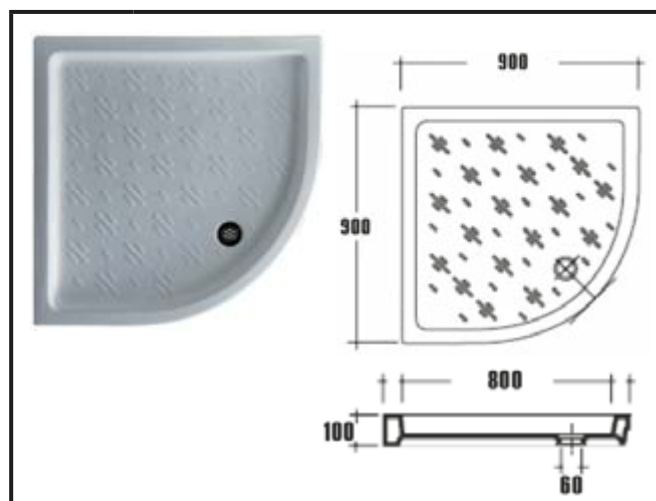
Š.Vokel Opis 1153008 TUŠ KADA KERAMIČKA 90x90 H=10 ART.1009
