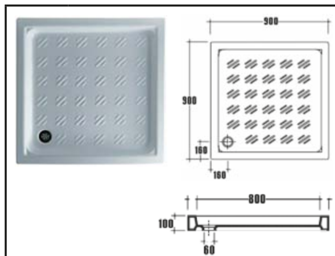
Š.Vokel Opis 1153006 TUŠ KADA KERAMIČKA 90x90 H=10 ART.1008
