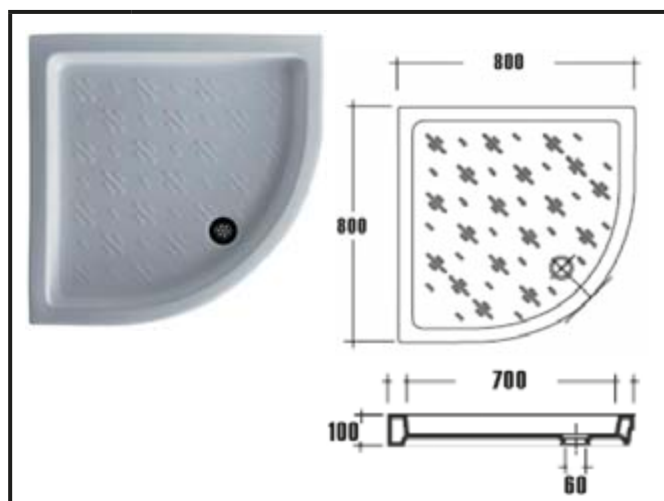
Š.Vokel Opis 1153007 TUŠ KADA KERAMIČKA 80x80 H=10 ART.1004
