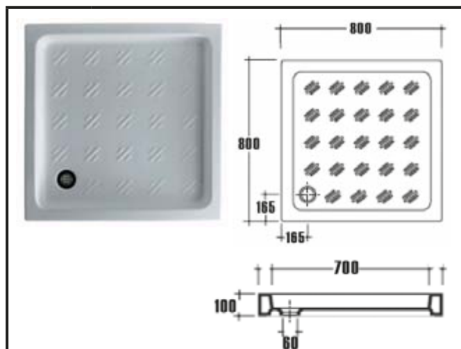
Š.Vokel Opis 1153005 TUŠ KADA KERAMIČKA 80x80 H=10 ART.1002
